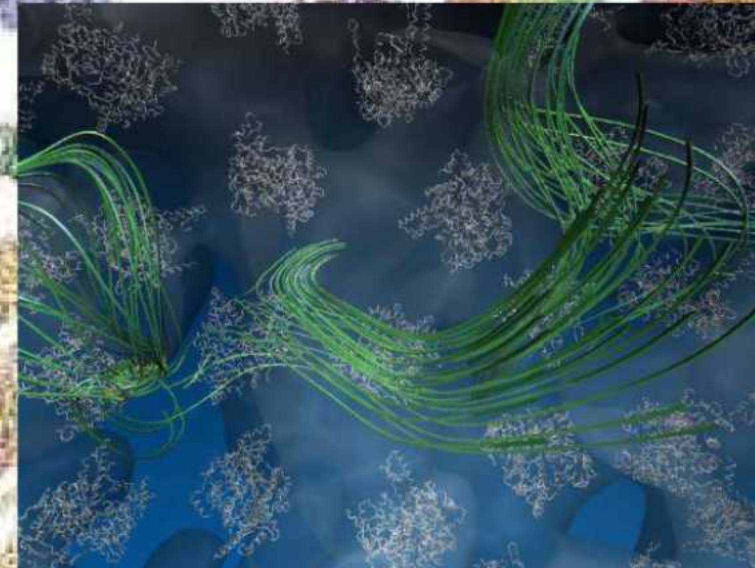
Lignes de courant dans la simulation d'une solution de protéines Streamlines in a multiprotein simulation
