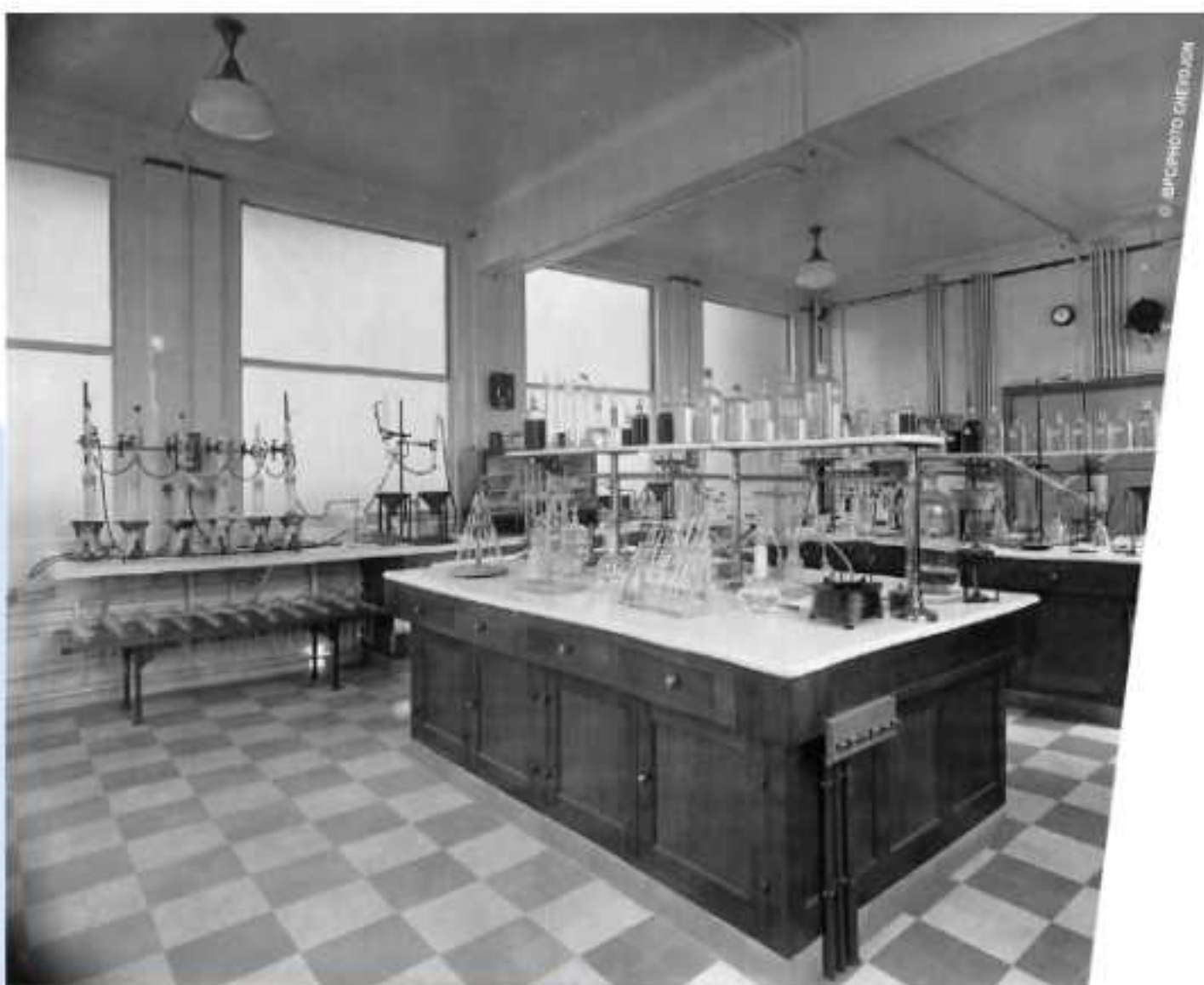
LABORATOIRE DE CHIMIE, 1 er ÉTAGE, 1930 CHEMISTRY LABORATORY, 1 st FLOOR, 1930
