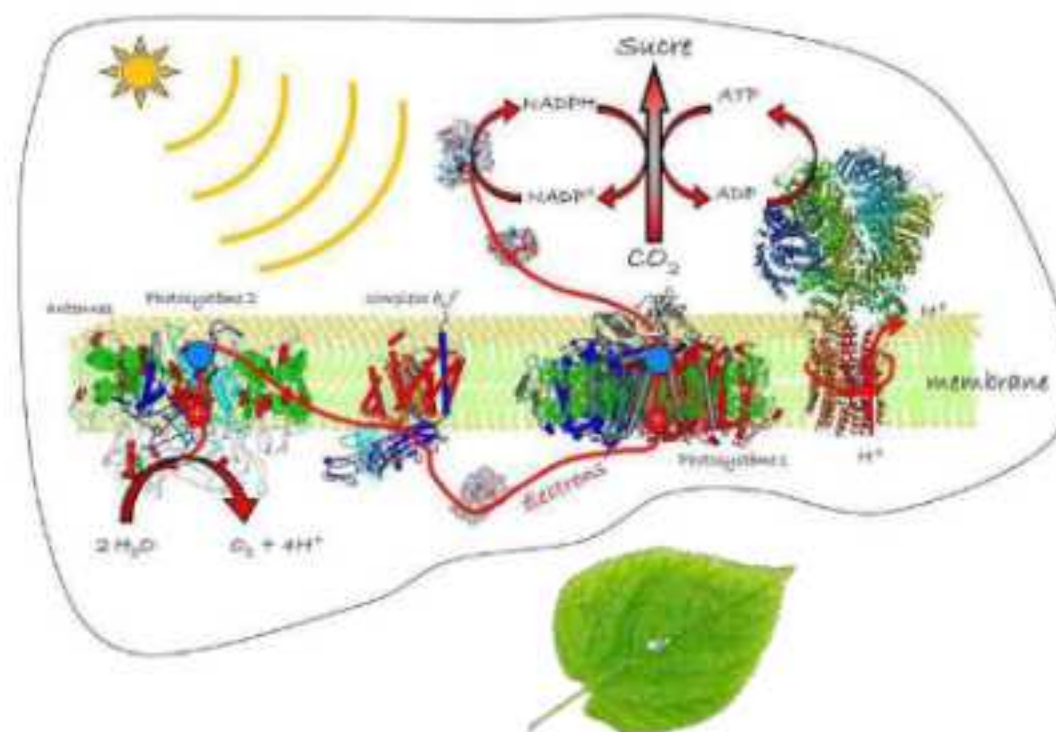
Schéma de la chaîne photosynthétique qui transforme la lumière en énergie chimique. Scheme of the photosynthetic chain that converts light into chemical energy.
