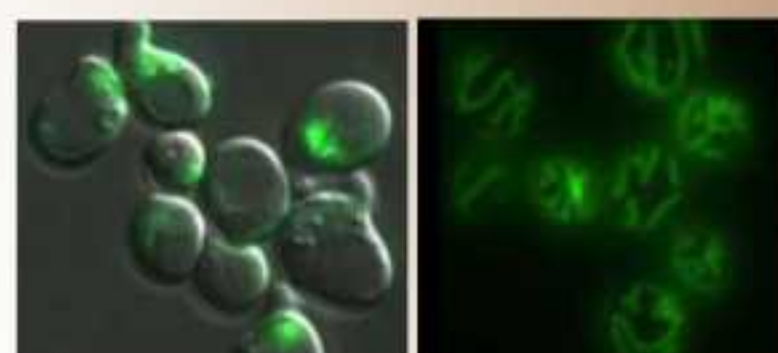
Marquage des mitochondries avec le fluorophore GFP visualisées au microscope optique à fluorescence.
