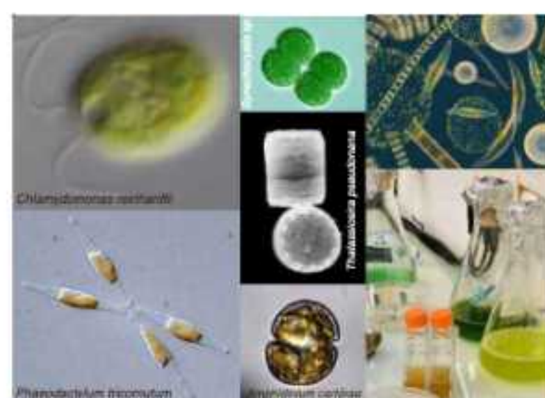
Organismes modèles utilisés au laboratoire Model organisms used in the laboratory
