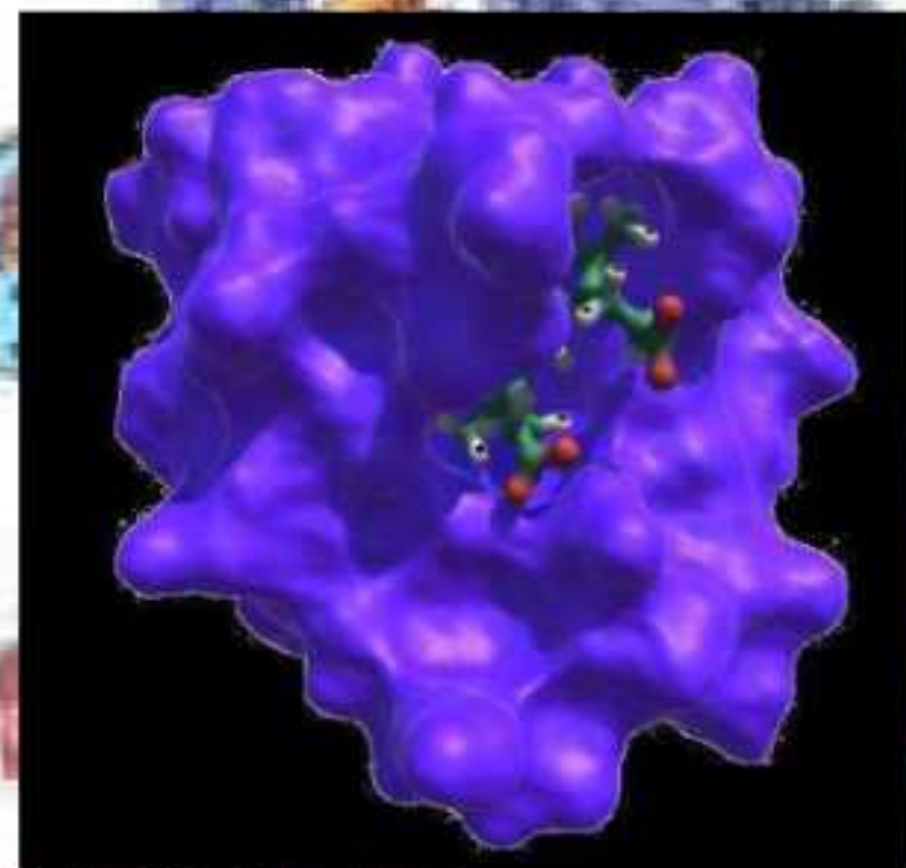
Ferrocyanide lié à l'hème Heme-bound ferrocyanide
