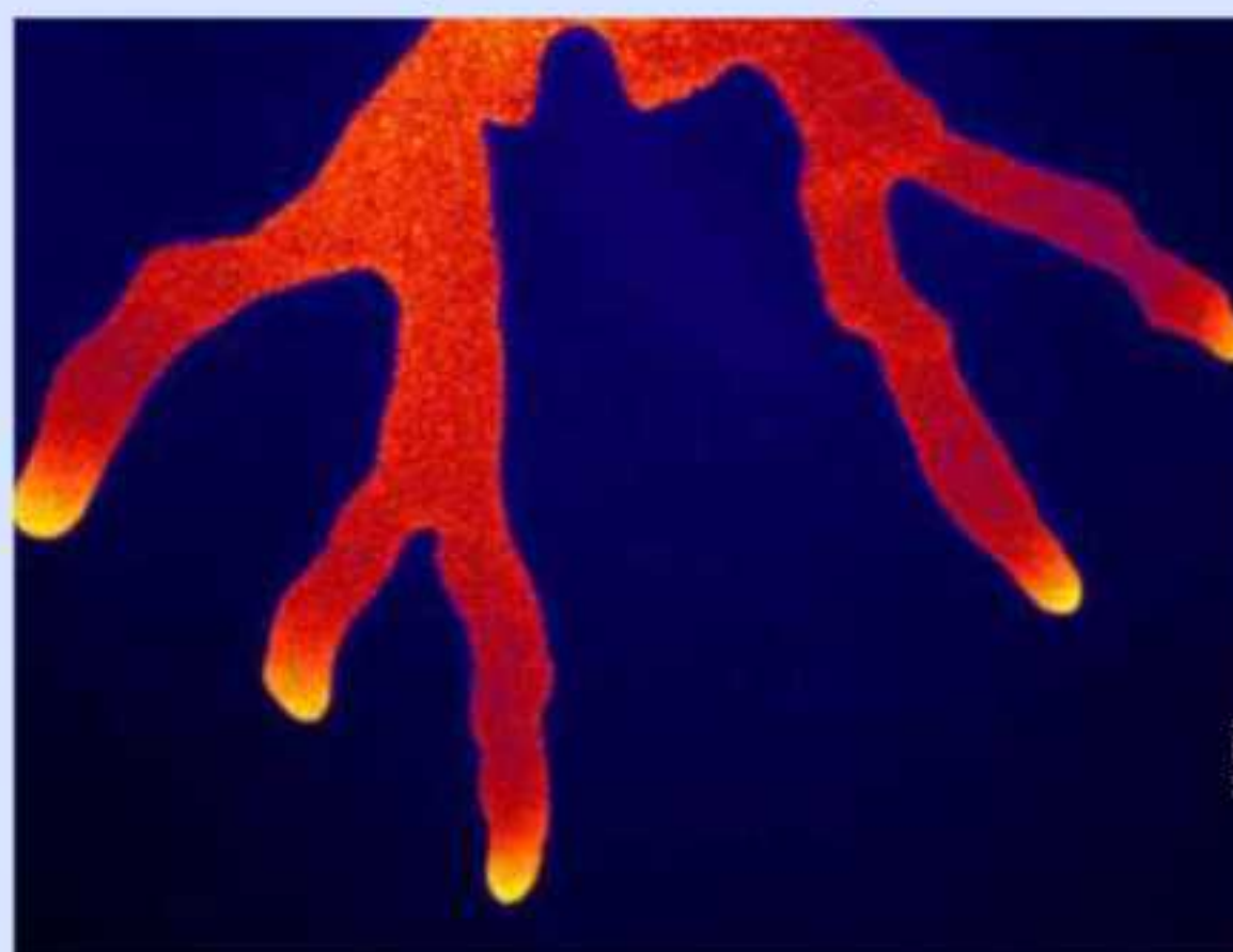
Une colonie migrante de Bacillus subtilis A swarming Bacillus subtilis colony (photo Harald Putzer)
